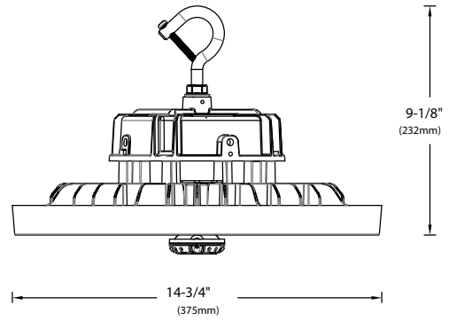
HCY28/HCY33
